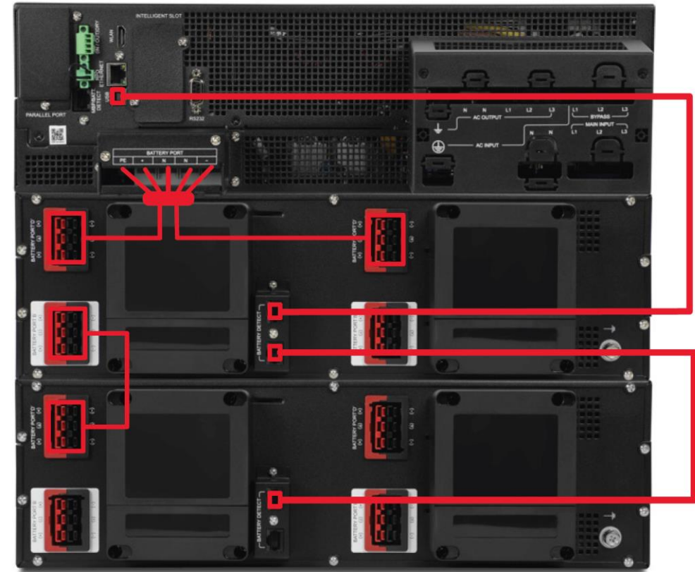
Схема подключения батарейного блока к ИБП
